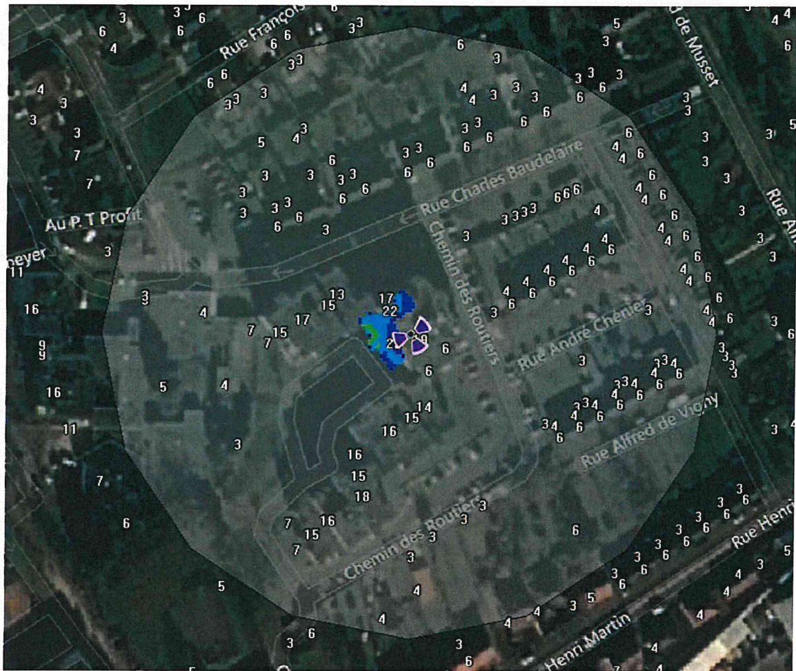
Fond de carte (photo aérienne), source : bing. Logiciel de simulation Cellerty, éditeur Orange Labs
